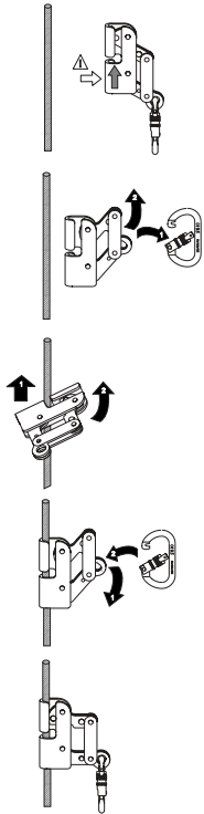
Mise en place sur le câble Setting-up on the cable
